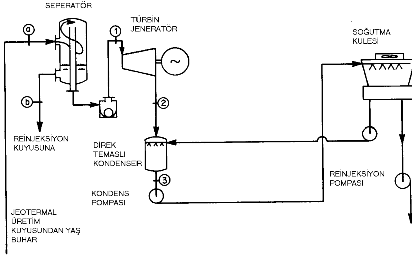
Şekil 2 Buhar ayırmalı (tek faz değişimli) bir santralin basitleştirilmiş şematik görünüşü
