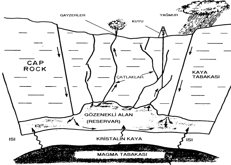
Şekil 1 Jeotermal – hidrotermal kaynak ve oluşumu için gerekli yapı
